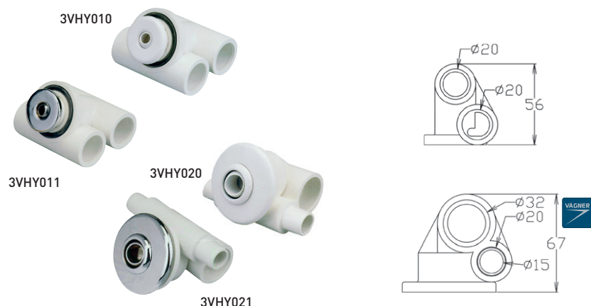
Osazení mikrotrysky přírubou pro fólii. Liner micronozzle fitted with flange.
